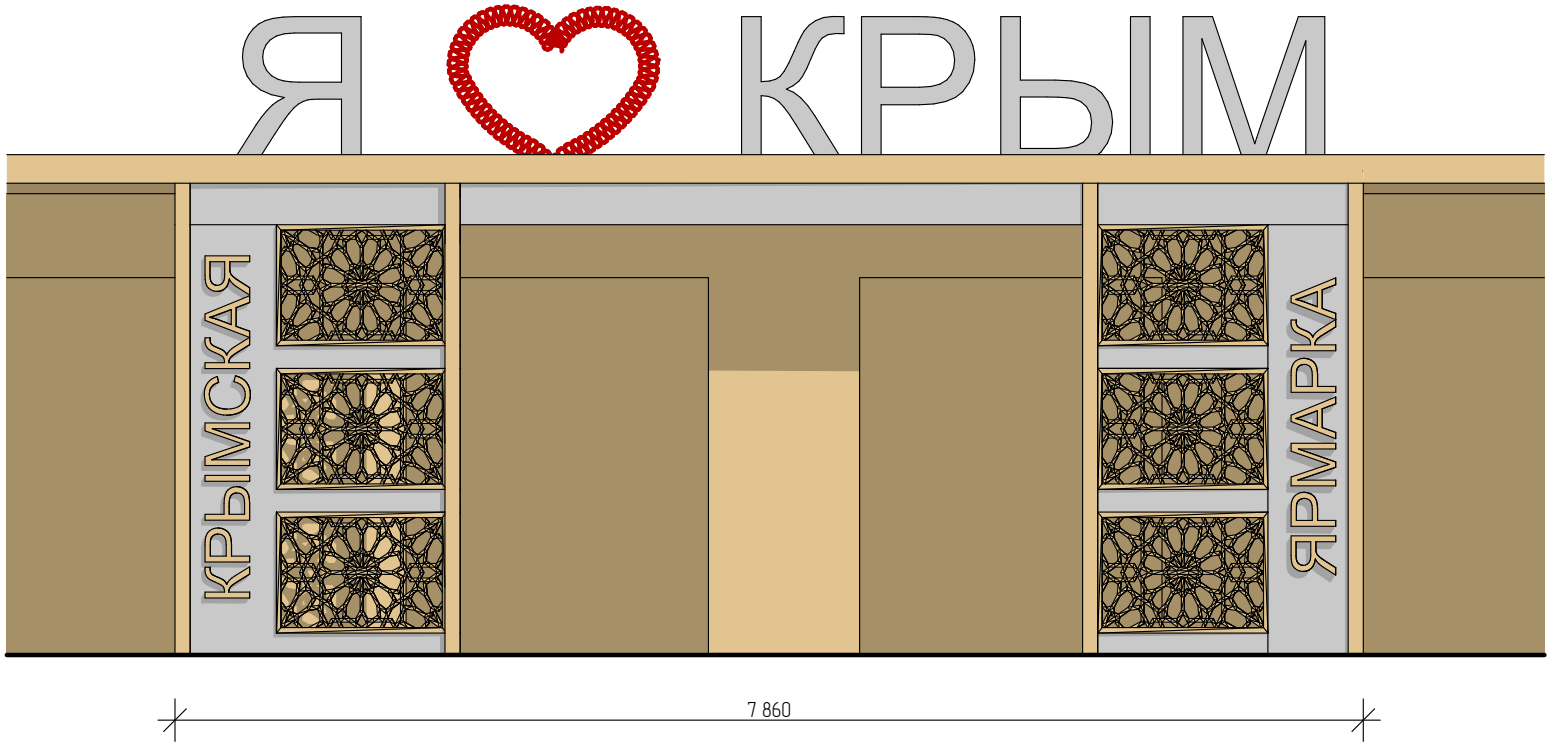
Фрагмент фасада М 1:50
